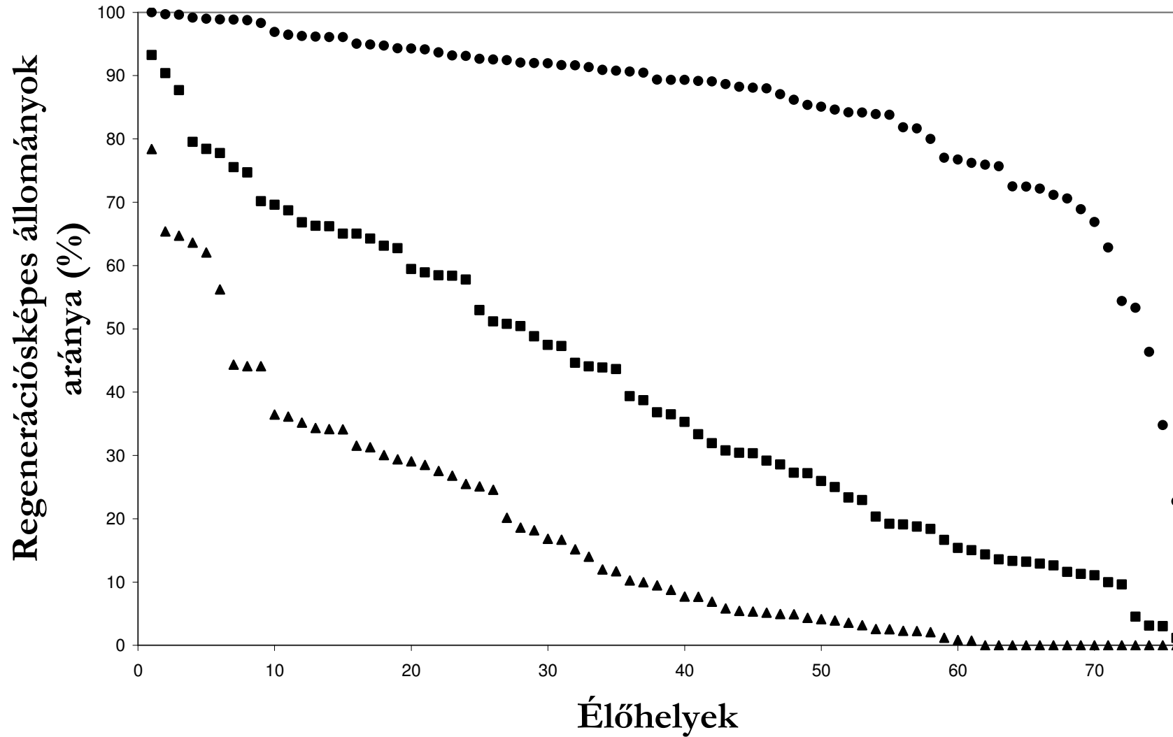
1. ábra. A grafikon az egyes vegetációtípusok regenerációs potenciáljainak országos átlagai csökkenő sorrendben (rang-korrelációs görbék). A legfelső görbe a helyben történő, a középső a szomszédos vegetációban való, az alsó görbe a parlagon történő regenerációt mutatja. Forrás: Seregélyes T., Molnár Zs., Bartha S., Csomós Á., Bölöni J. (2008): A hazai növényzet regenerációs képessége a MÉTA adatbázis adatai alapján. IV. Magyar Földrajzi Konferencia előadaskötete, Debrecen, pp. 219-229.
