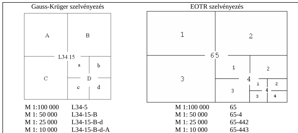
1. ábra: A Gauss-Krüger és az EOTR szelvényezés (Forrás: Magyarai 2007)
